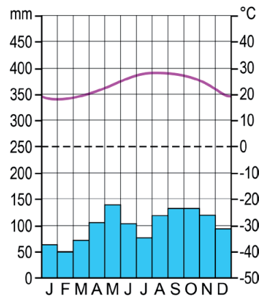
klimaatdiagram b
