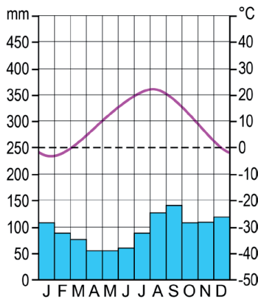
klimaatdiagram a
