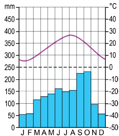
klimaatdiagram d
