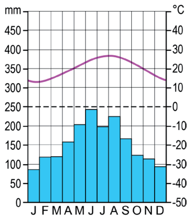
klimaatdiagram c
